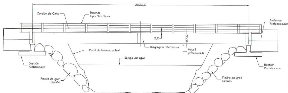
Sección longitudinal propuesta por el contratista
